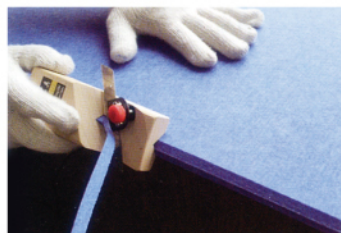
◆ 利用倒角器開始45°倒角 Chamfer 45° bevel edge chamfering tool.
