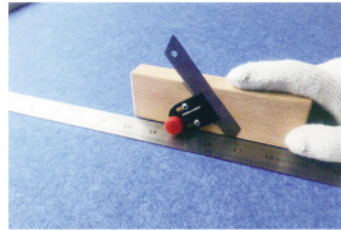
◆ 固定硬性靠尺，不要完全切斷 Cut 4/5 depth of the panel.
